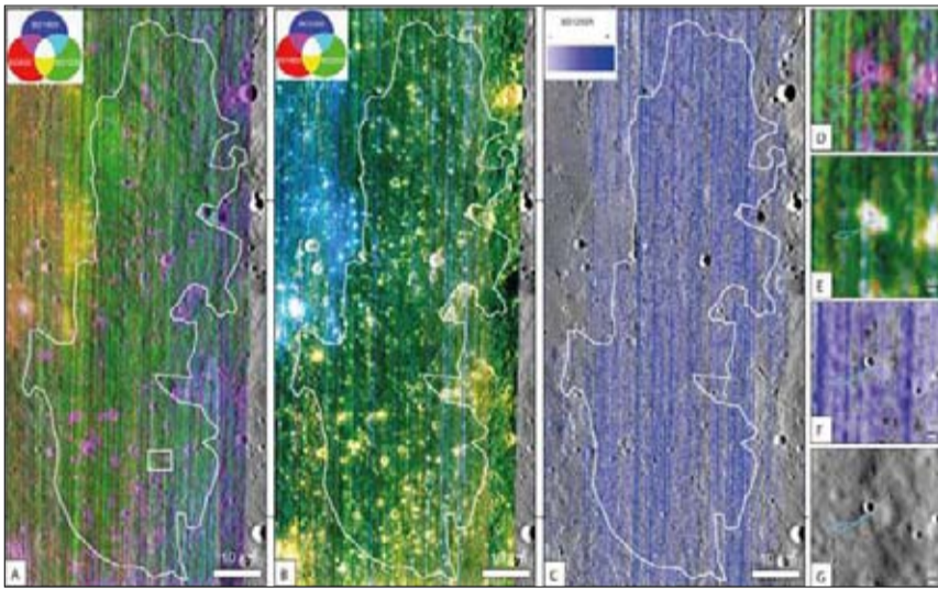
يتيح التحليل الطيفي للتربة القمرية تحديد المعادن المختلفة التي تتكون منها الصخور
