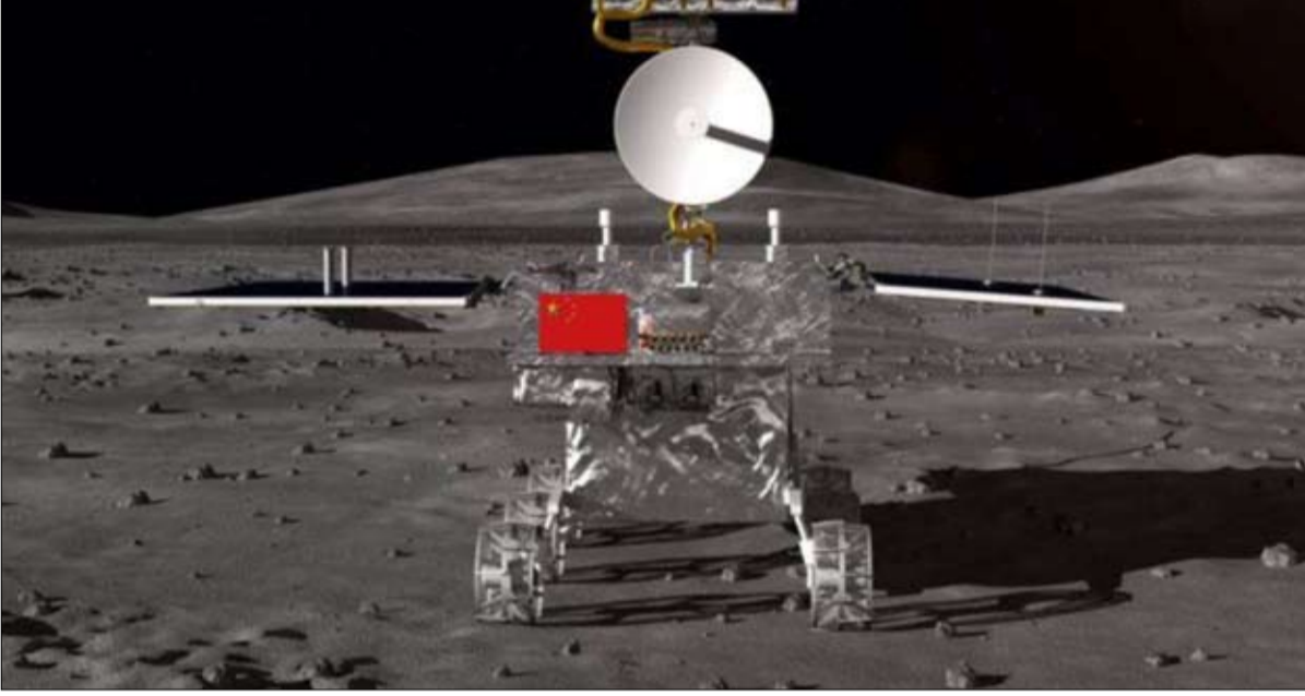
هبوط المركبة الصينية تشانغ أه 4 على الجانب البعيد من القمر
